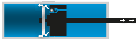
Cofanie amortyzatora
